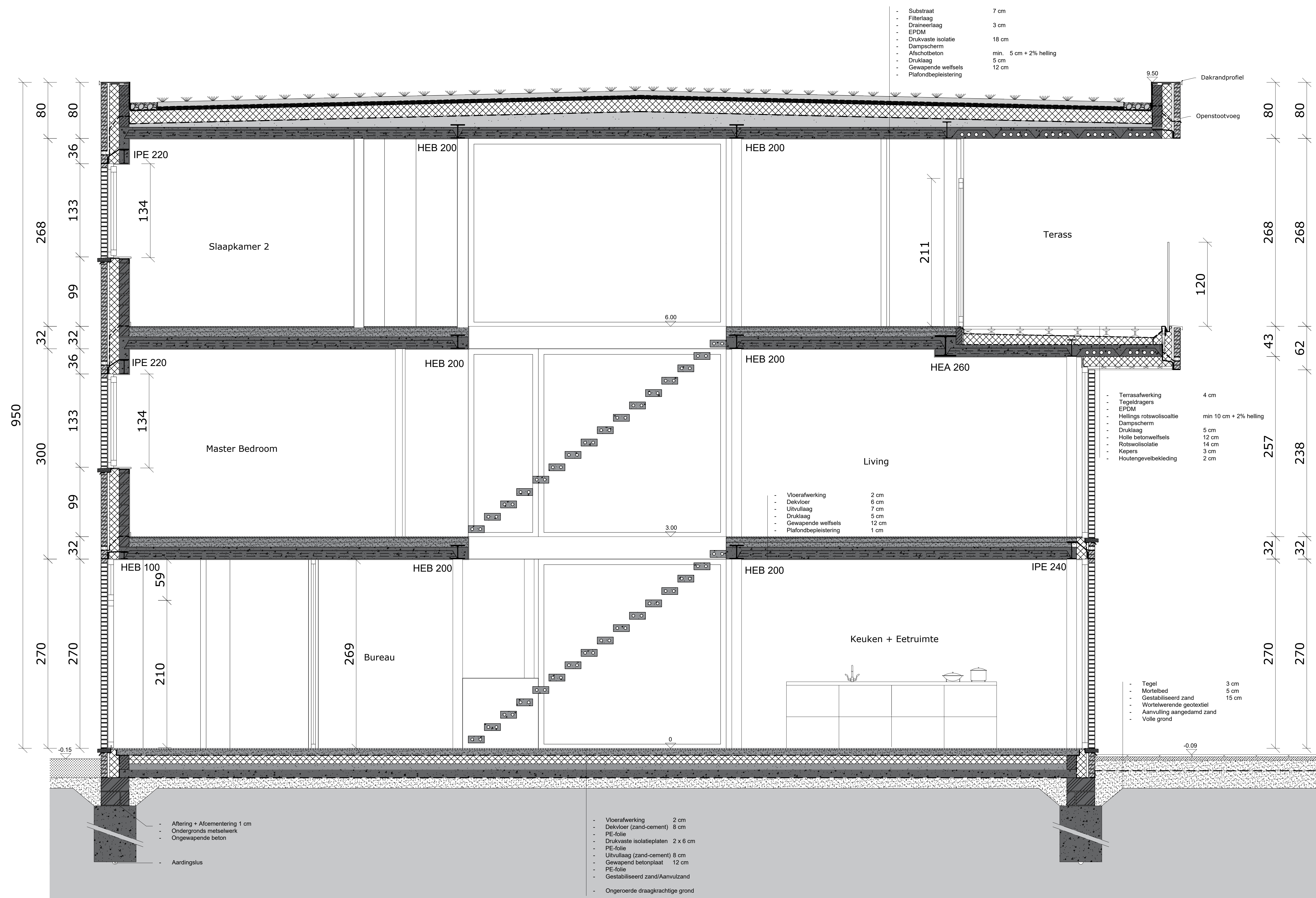
Doorsnede AA' 1:25
