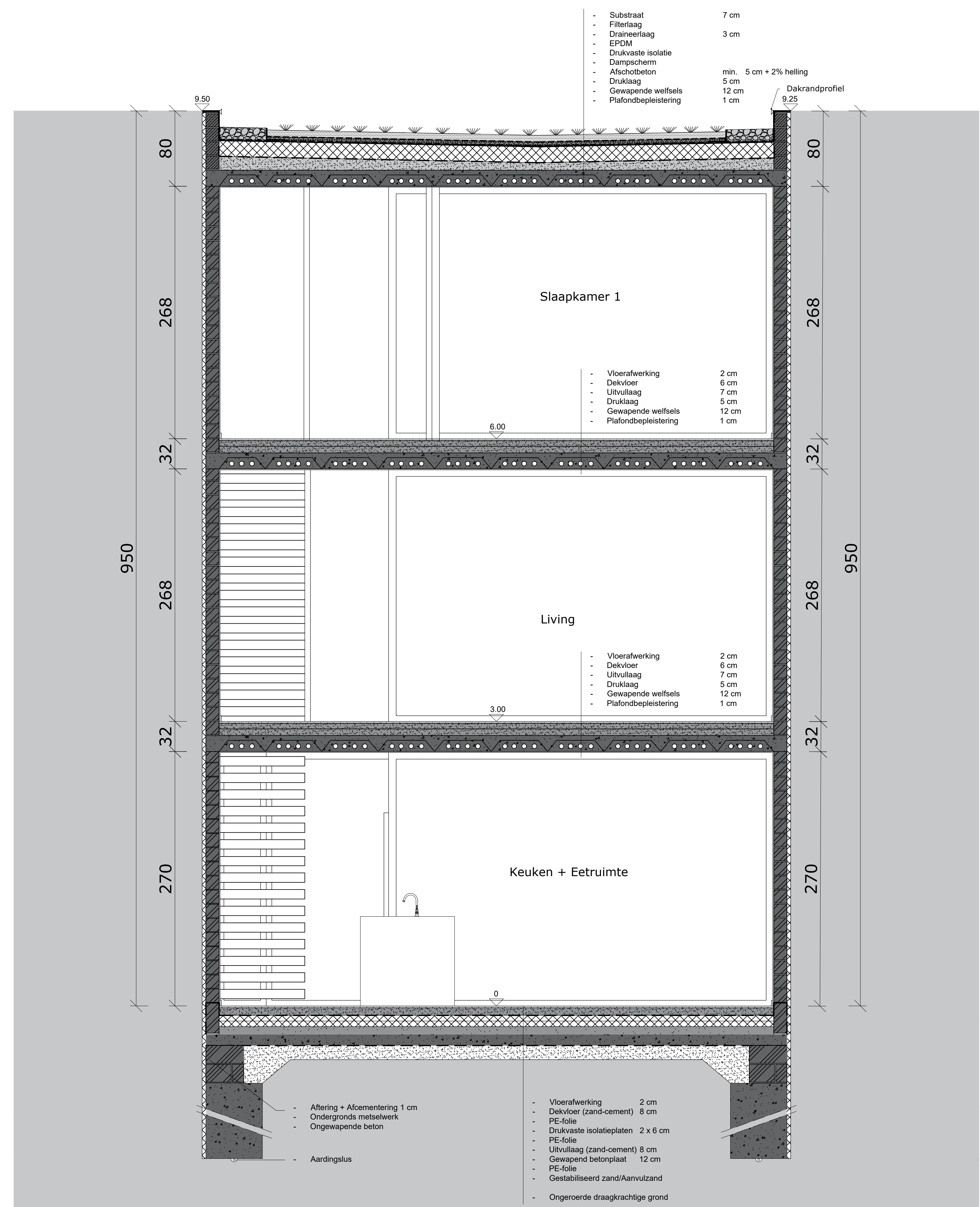
Doorsnede BB' 1:25
