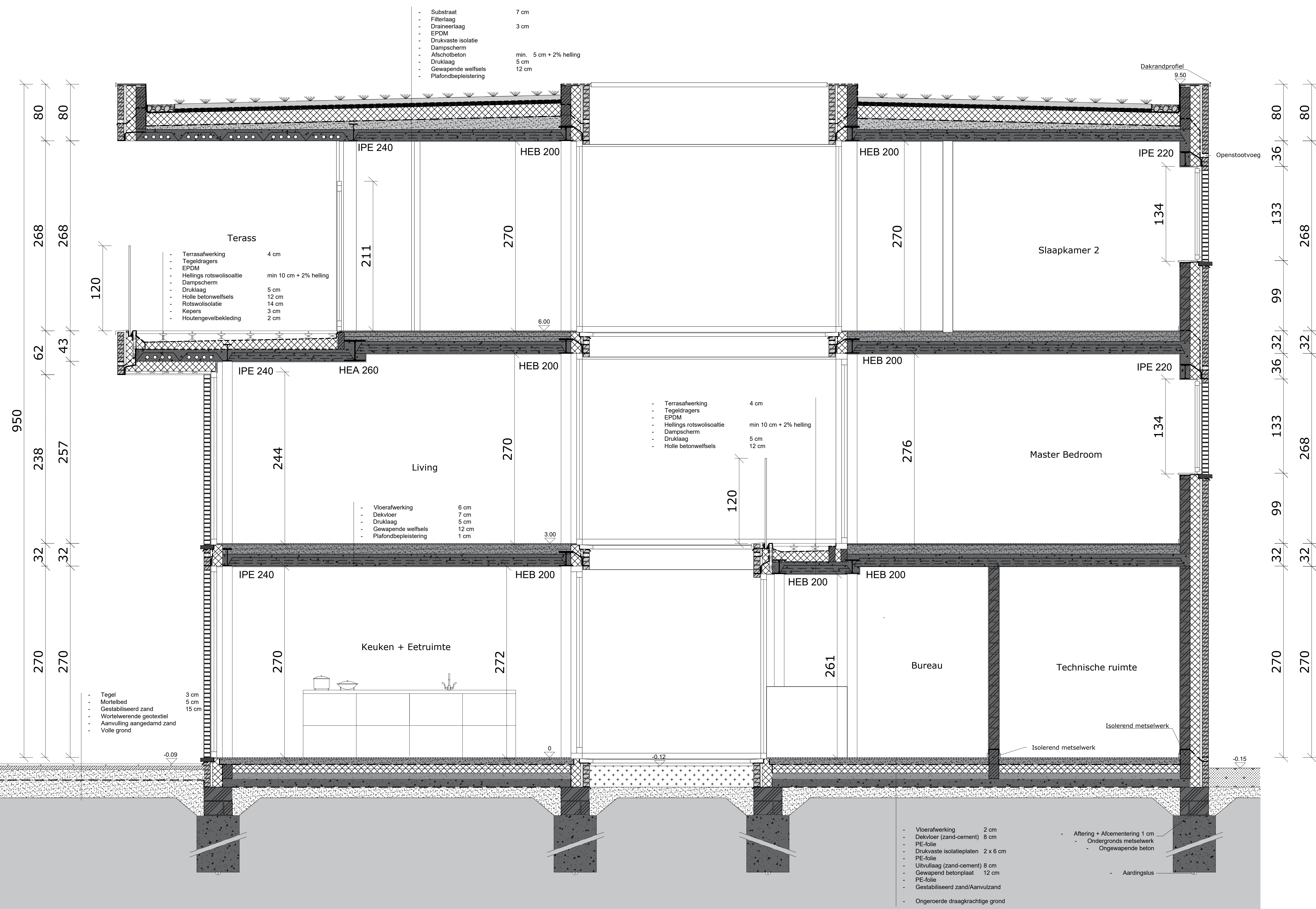
Doorsnede CC' 1:25
