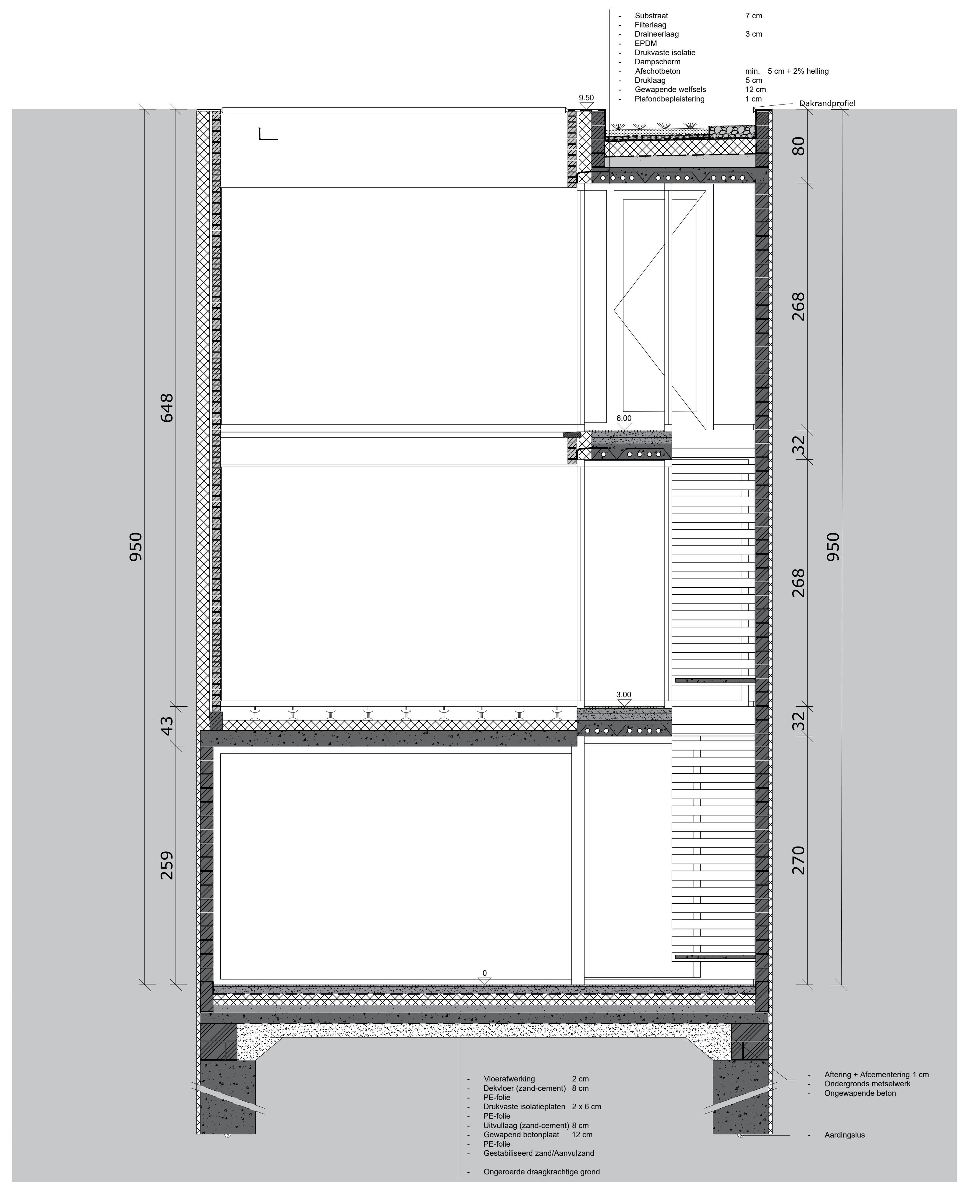
Doorsnede DD' 1:25
