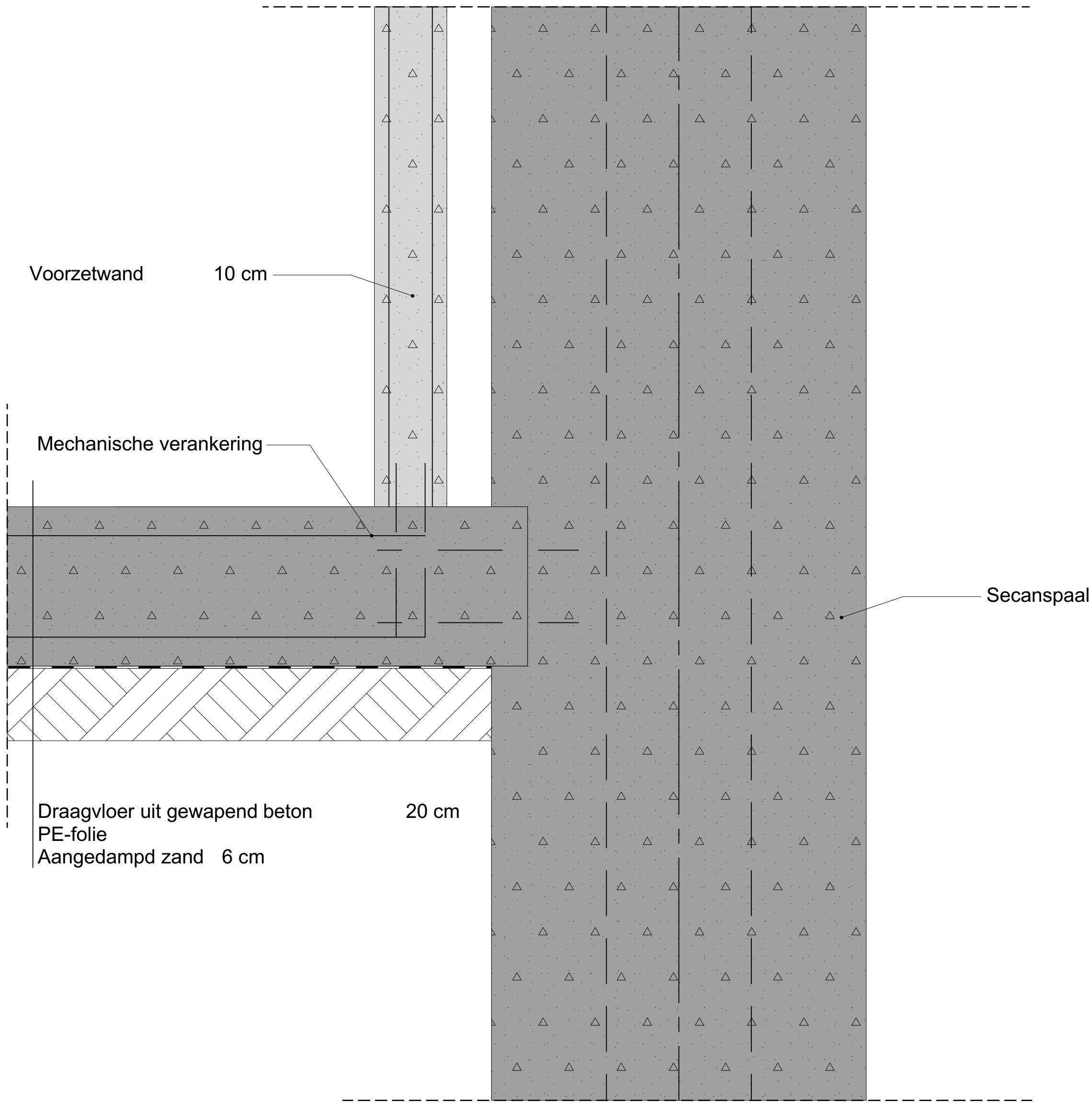
Detail kelder met secanspalen+
