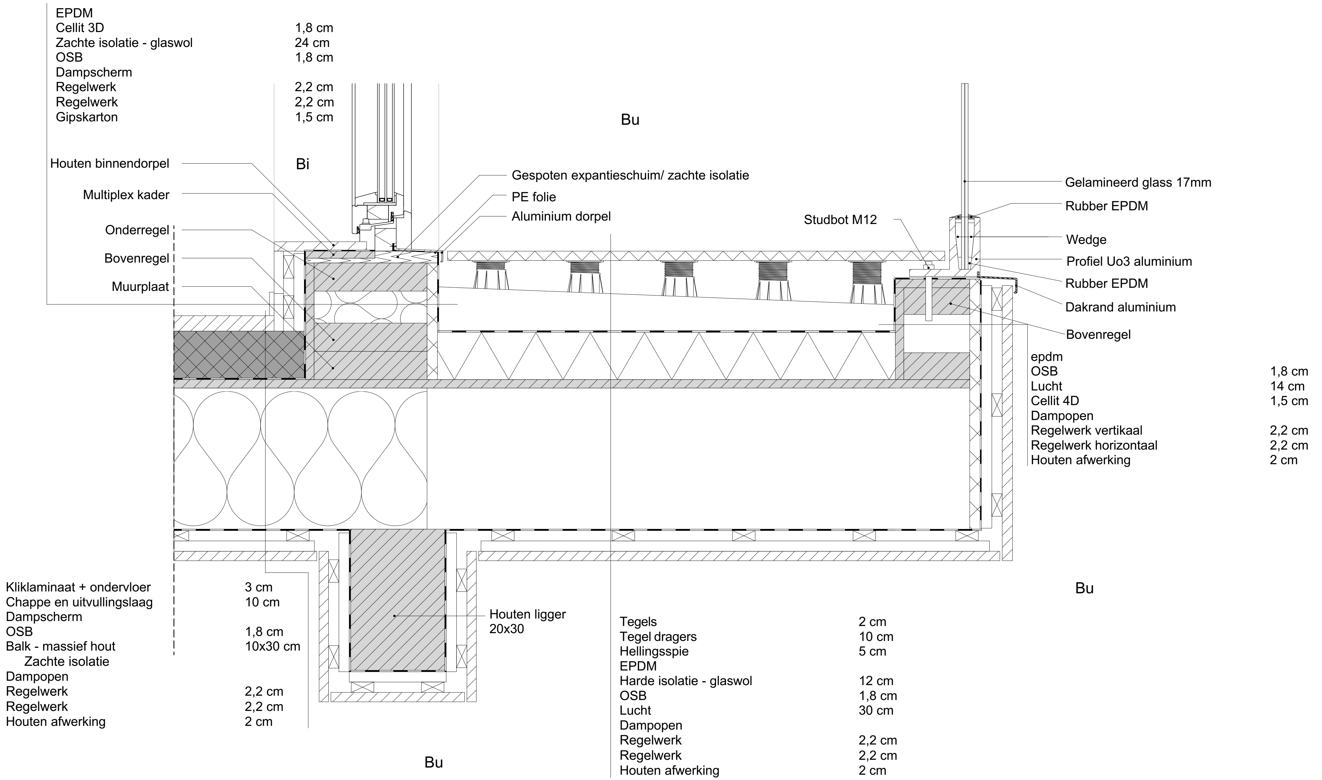
Detail buitenmuur op vloerplaat met terras
