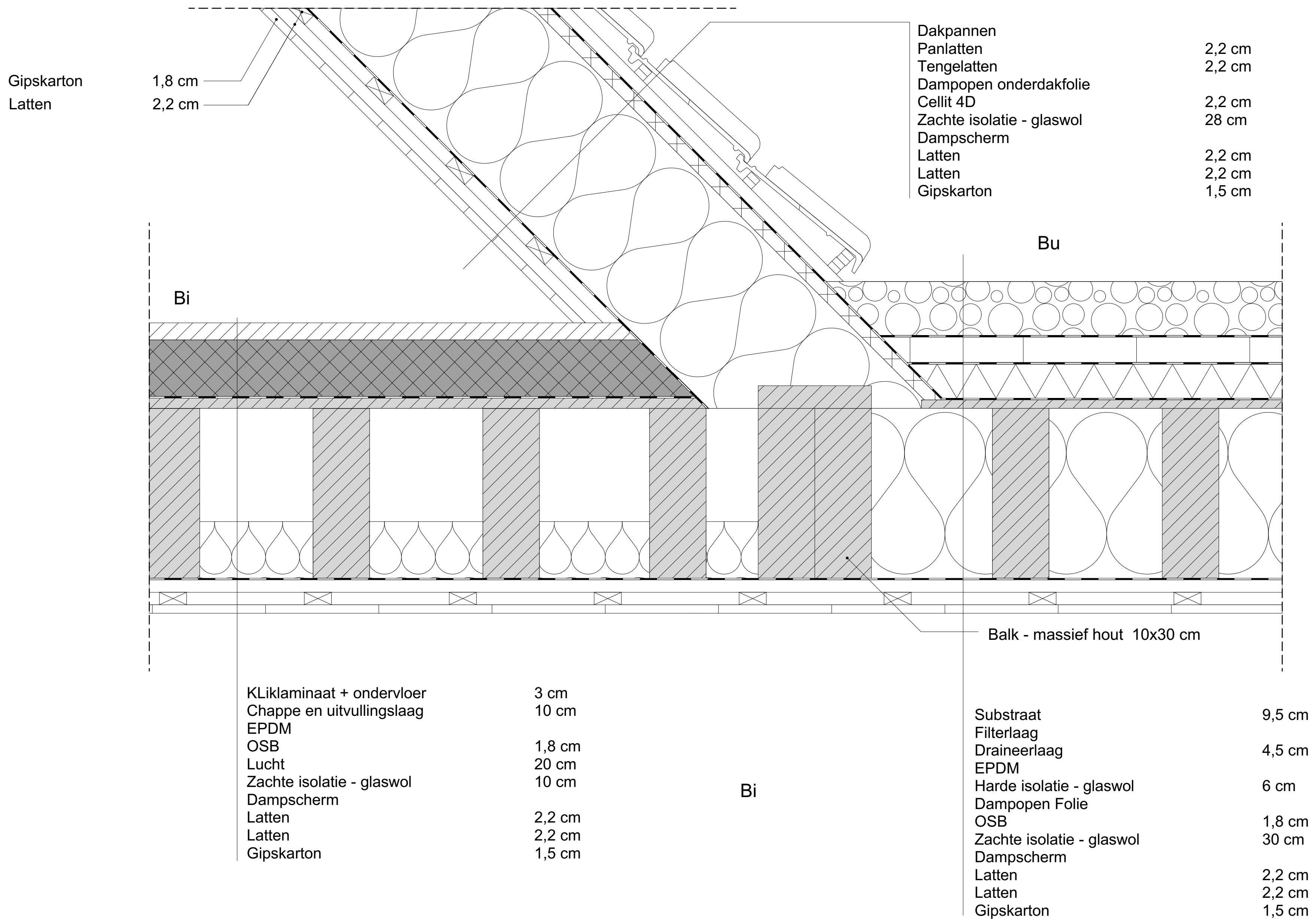
Detail Dak op vloerplaat en groendak
