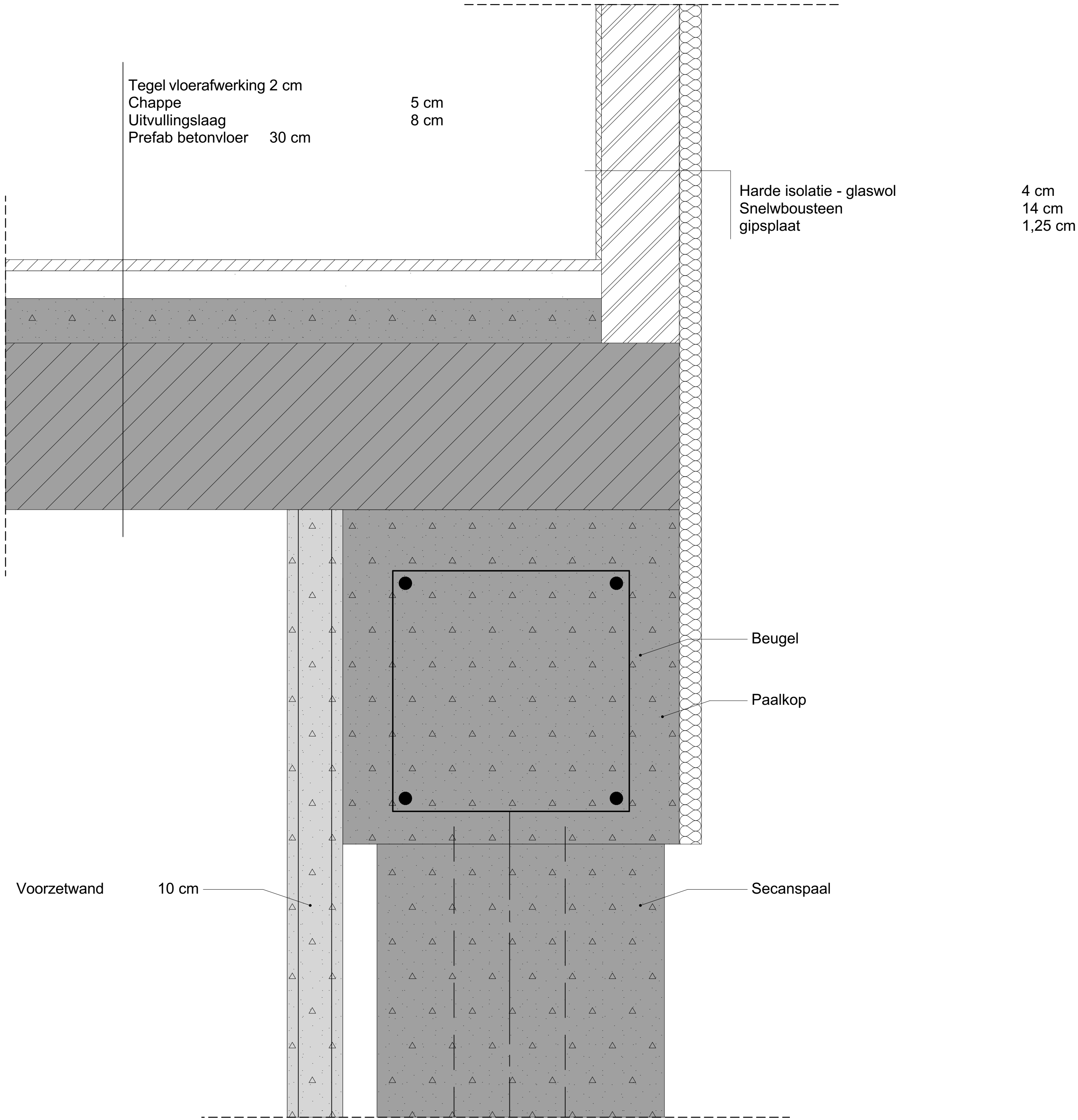
Detail Gelijkvloers op secanspalen+
